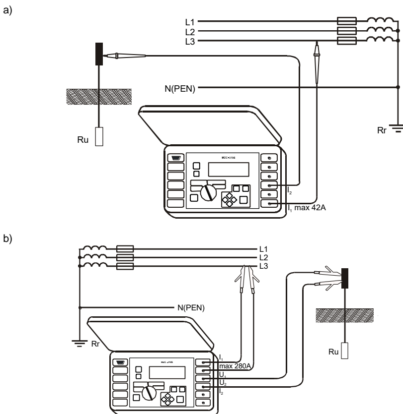
Ilustración22. La manera de la conexión del medidor MZC-310S en el caso de las mediciones de la resistencia de las tomas de tierra a la red TN-C, TN-S y TT: a) por medio del método de dos polos b) por medio del método de cuatro polos
