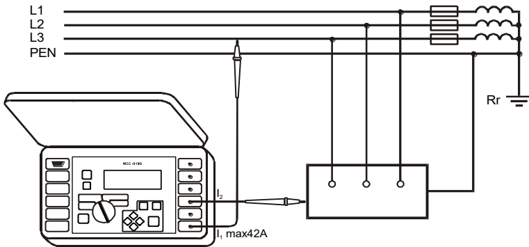
Ilustración15. Medición de la impedancia en el circuito de trabajo (L-L) por medio del método de cuatro polos
